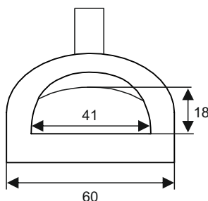
Sezione frontale
