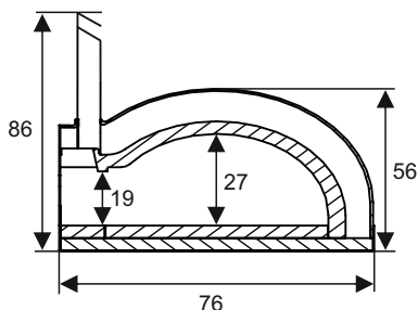
Sezione trasversale
