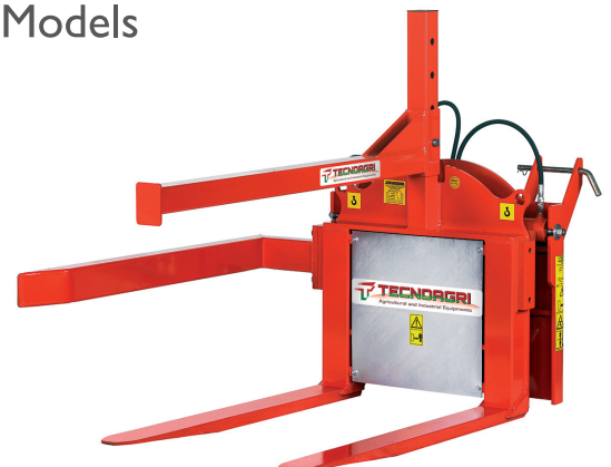
Rovesciatore Idraulico Braccio Meccanico Hydraulic Side-Tipper Mechanical Arm
