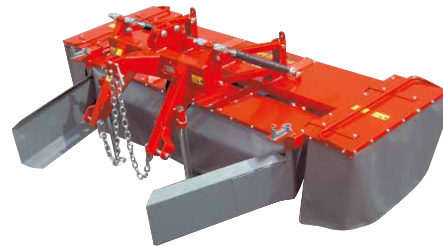
FALCIATRICE/FALCIACONDIZIONATRICE FRONTALE FR/G315 Faucheuse-conditionneuse frontal FR/G315
