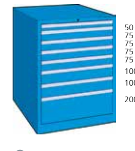
● h. 850 mm • 8 cassetti G85 81 estrazione parziale G85 81V estrazione totale 75 kg
