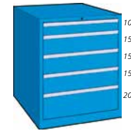
● h. 850 mm • 5 cassetti M85 51 estrazione parziale M85 51T estrazione totale 200 kg M85 51V estrazione totale 75 kg
