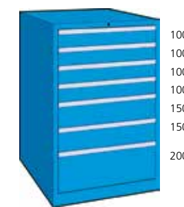
● h. 1000 mm • 7 cassetti G100 71 estrazione parziale G100 71V estrazione totale 75 kg
