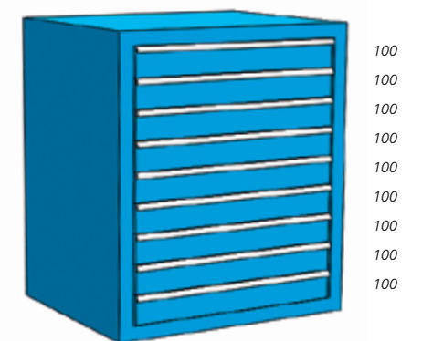
● h. 1000 mm • 9 cassetti S100 01 estrazione parziale 100 kg S100 02V estrazione totale 75 kg S100 02T estrazione totale 200 kg
