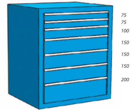
● h. 1000 mm • 7 cassetti S100 71 estrazione parziale 100 kg S100 71V estrazione totale 75 kg S100 71T estrazione totale 200 kg
