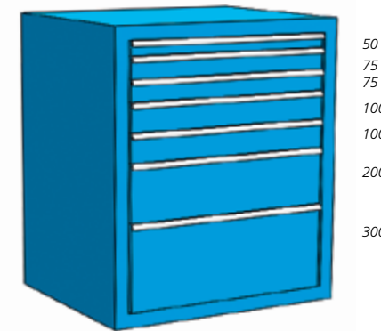
● h. 1000 mm • 7 cassetti S100 74 estrazione parziale 100 kg S100 74V estrazione totale 75 kg S100 74T estrazione totale 200 kg
