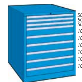
● h. 850 mm • 9 cassetti M85 91 estrazione parziale M85 91T estrazione totale 200 kg M85 91V estrazione totale 75 kg
