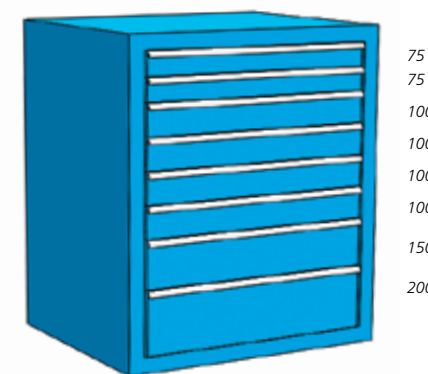
● h. 1000 mm • 8 cassetti S100 88 estrazione parziale 100 kg S100 88V estrazione totale 75 kg S100 88T estrazione totale 200 kg
