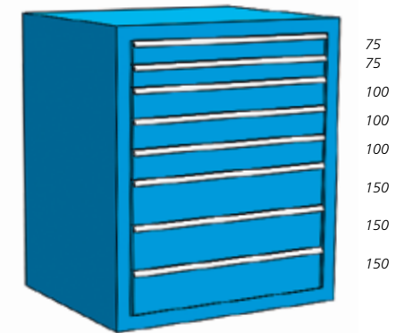
● h. 1000 mm • 8 cassetti S100 05 estrazione parziale 100 kg S100 05V estrazione totale 75 kg S100 05T estrazione totale 200 kg
