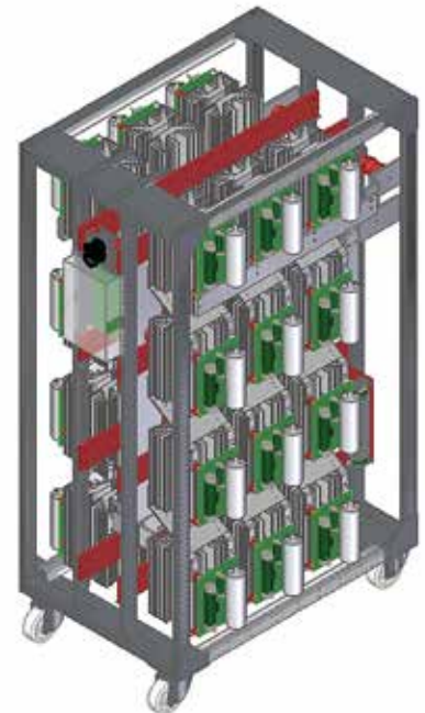
Redresseur au silicium monté sur châssis roulant pour sous-stations ferroviaires RFI 3,6 kV, 5,4 MW
