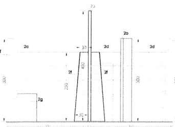
elevation D-D'
