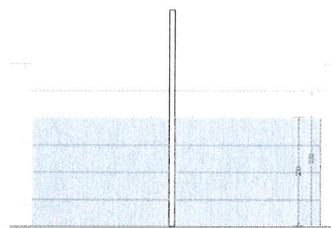
elevation B-B'
