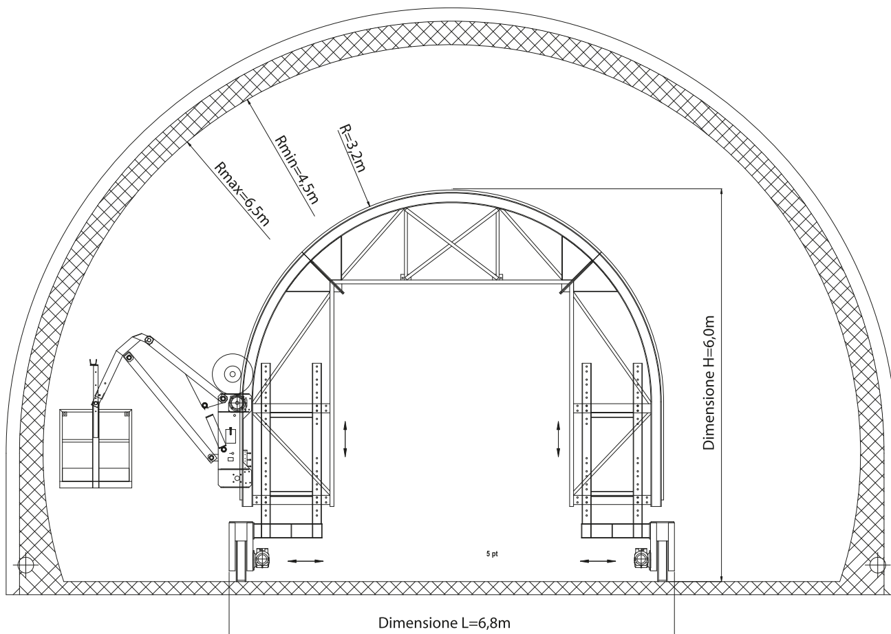
LAY-OUT generale/General LAY-OUT/LAY-OUT générale
