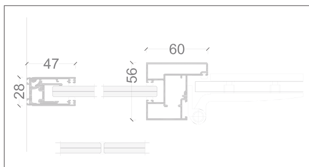
HORIZONTAL SECTION GLASS DOOR
