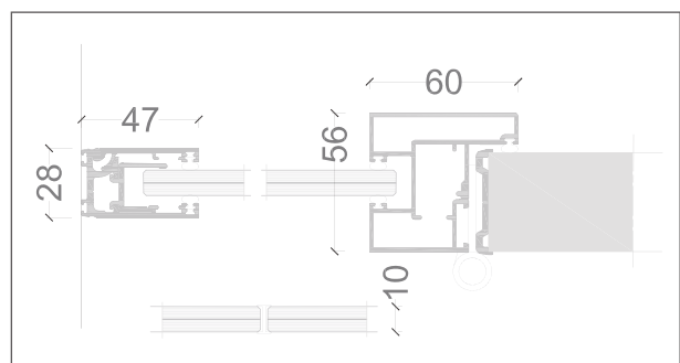
HORIZONTAL SECTION WOOD DOOR
