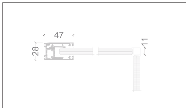
90° ANGLE
