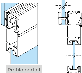
Door profile 1 | Perfil puerta 1
