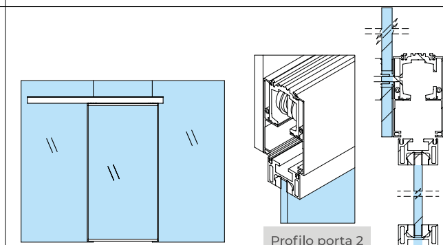
Door profile 2 | Perfil puerta 2
