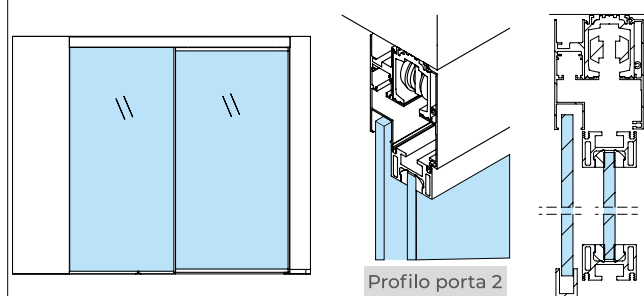
Door profile 2 | Perfil puerta 2
