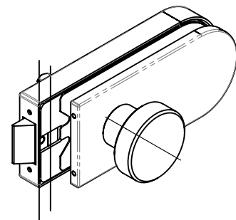
Serratura orizzontale Horizontal lock Cerradura horizontal
