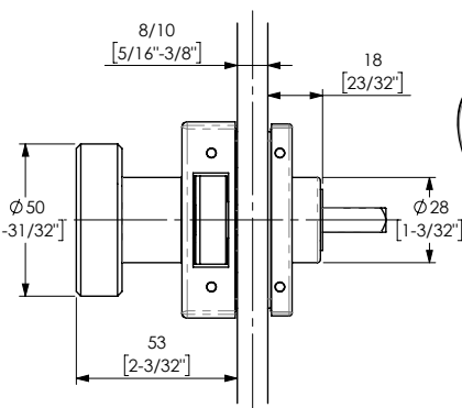
Serratura orizzontale Horizontal lock Cerradura horizontal
