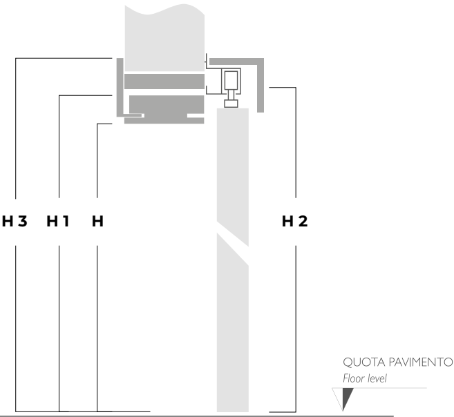
Apertura Destra Right opening
