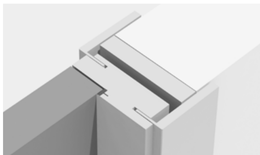
Sezione porta a battente con cerniere a scomparsa
