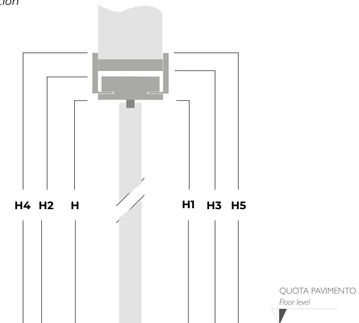
Apertura Destra Right opening
