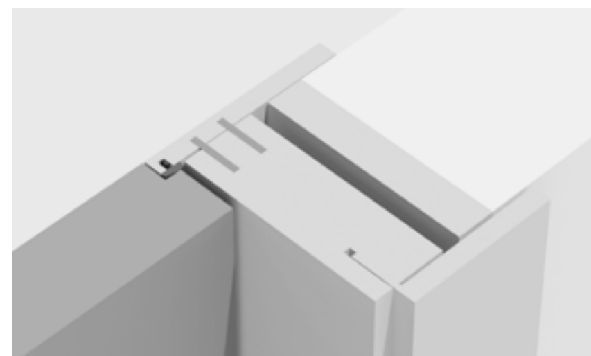
Sezione porta complanare con apertura inversa
