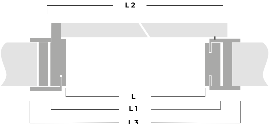
Sezione verticale Vertical section
