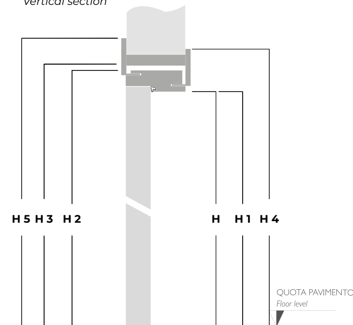
Sezione verticale Vertical section
