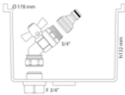
Pozzetto con rubinetto idrante intercambiabile con valvola a sfera, completo di raccordo rapido Shut-off box with interchangeable ball valve hydrant faucet, complete with quick connector
